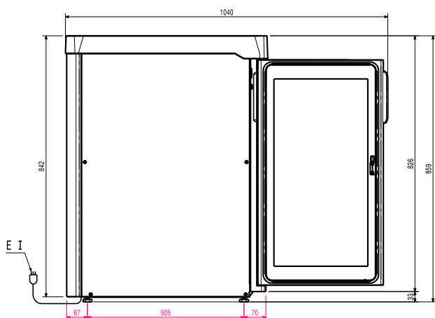
Zij aanzicht
